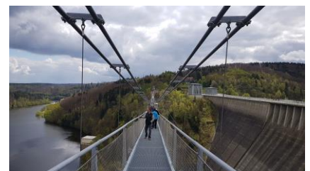
Hängebrücke an der Rappodetalsperre
